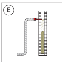
Kerndämmung
