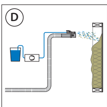
Feuchtsprühen
